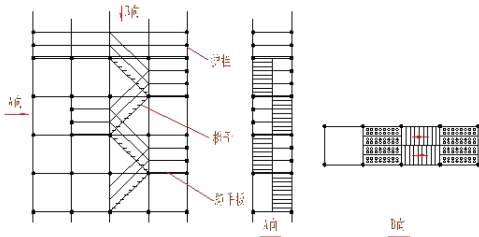
图 6.1.12 人行梯架设置示意图
